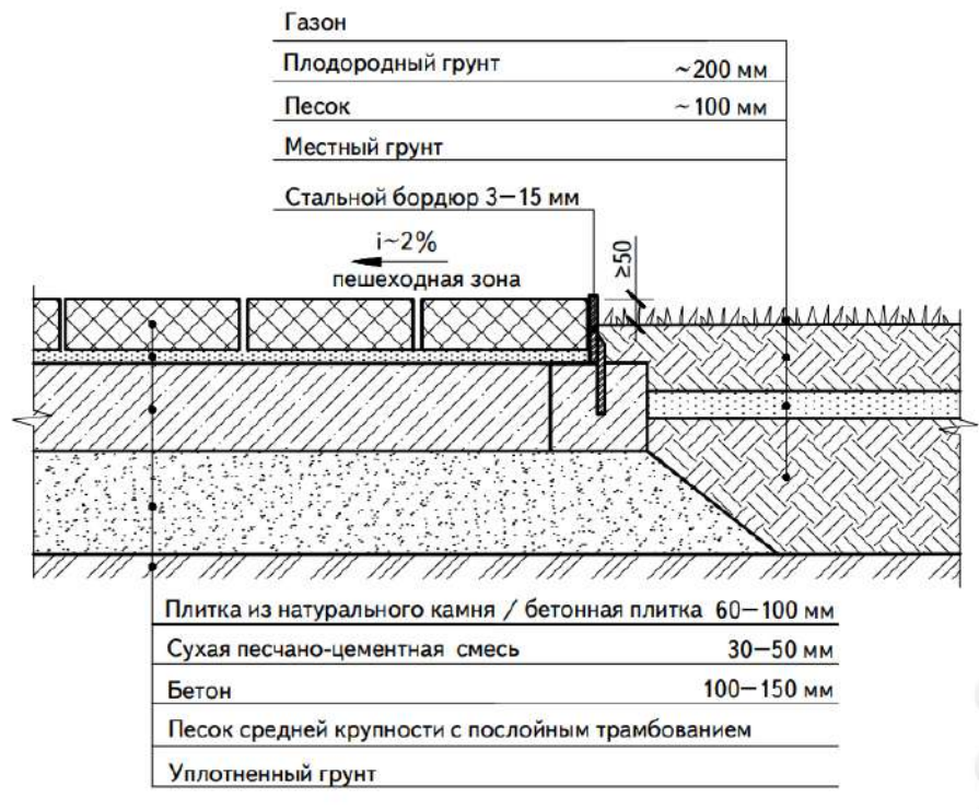
илл. 1.2.4. ПРИНЦИПИАЛЬНАЯ СХЕМА СОПРЯЖЕНИЯ ПЕШЕ- ХОДНОЙ ЗОНЫ ИЗ БЕТОННОЙ ПЛИТКИ (ПЛИТКИ ИЗ НАТУ- РАЛЬНОГО КАМНЯ) И ГАЗОНА ЧЕРЕЗ СТАЛЬНОЙ БОРДЮР
