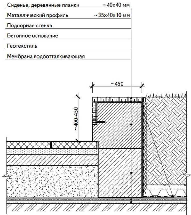
Илл. 5.1.3. Принципиальная схема устройства сиденья на подпорной стене
