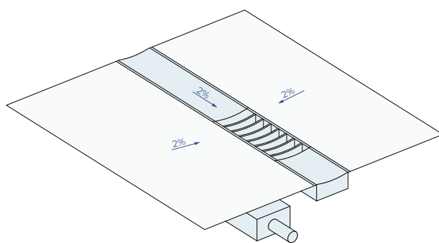
линейный водоотвод
