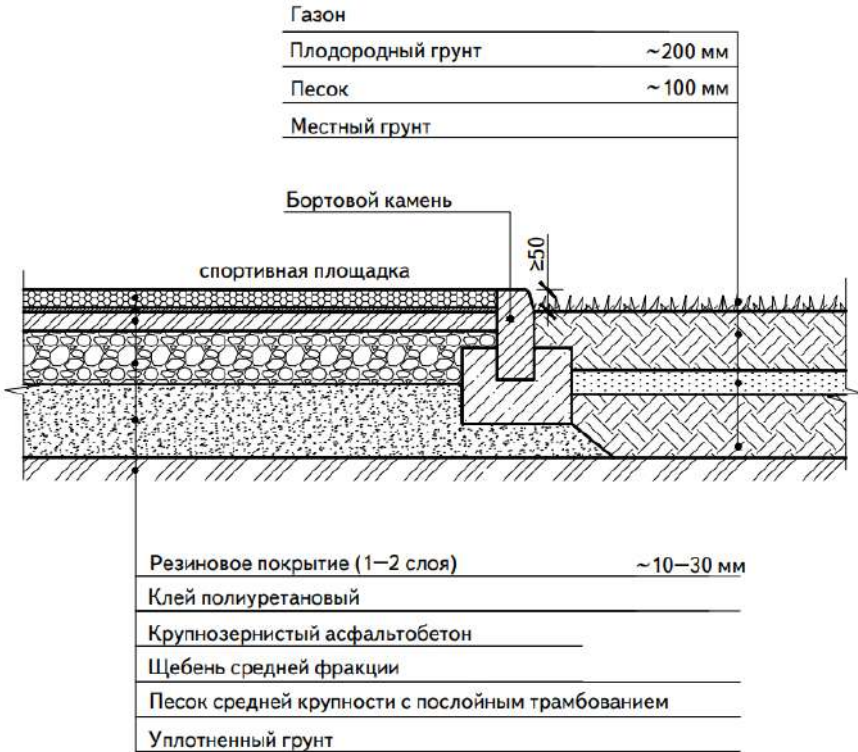
Илл. 1.2.6. ПРИНЦИПИАЛЬНАЯ СХЕМА СОПРЯЖЕНИЯ СПОРТИВНОГО ПОКРЫТИЯ И ГАЗОНА
