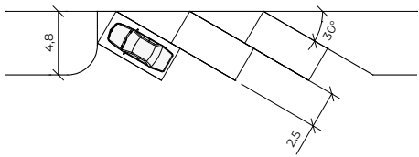
Илл. 6.2.4. расстановка парковочных мест под углом 30°
