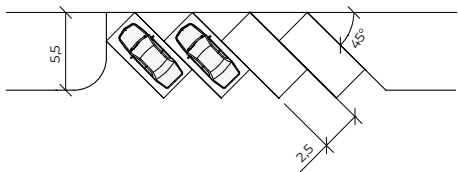
Илл. 6.2.5. расстановка парковочных мест под углом 45°
