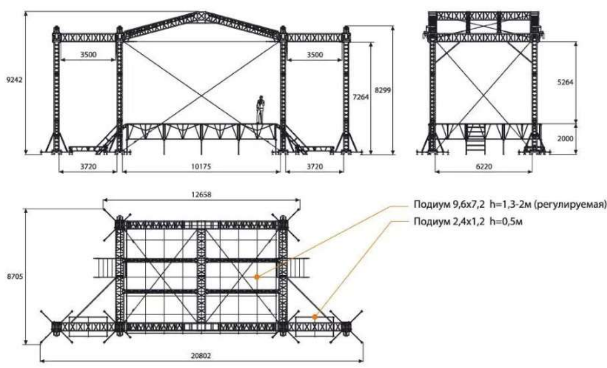
Илл. 5.6.3. ПРИНЦИПИАЛЬНАЯ СХЕМА МОНТАЖА СБОРНО-РАЗБОРНОЙ СЦЕНЫ
