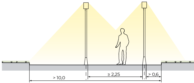
Илл. 3.7. ДВУХРЯДНАЯ ПРЯМОУГОЛЬНАЯ СХЕМА РАСПОЛОЖЕНИЯ ОПОР ОСВЕЩЕНИЯ
