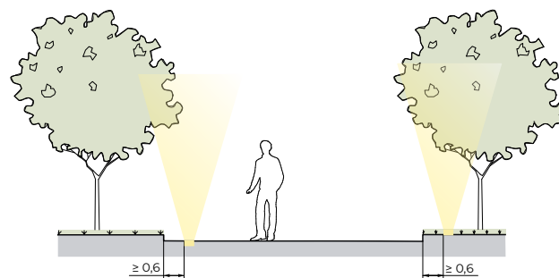
ИЛЛ. 2.12. ОСВЕЩЕНИЕ, ВСТРОЕННОЕ В МОЩЕНИЕ
