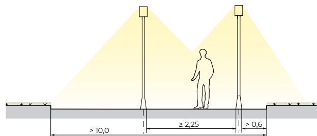
Илл. 6.13. ДВУХРЯДНАЯ ПРЯМОУГОЛЬНАЯ СХЕМА РАСПОЛОЖЕНИЯ ОПОР ОСВЕЩЕНИЯ
