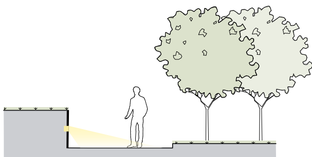
Илл. 2.13. ОСВЕЩЕНИЕ, ВСТРОЕННОЕ В ПОДПОРНУЮ СТЕНКУ
