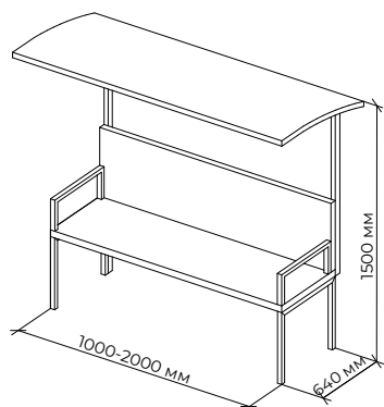
Скамья с навесом
