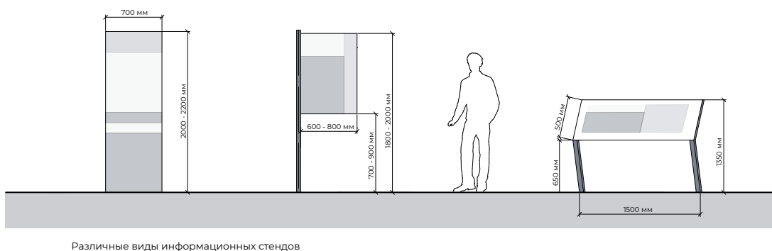
Илл. 5.7.4. ГАБАРИТЫ ОБОРУДОВАНИЯ ДЛЯ НАВИГАЦИИ
