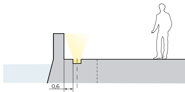
Светильник, встроенный в покрытие береговой зоны
