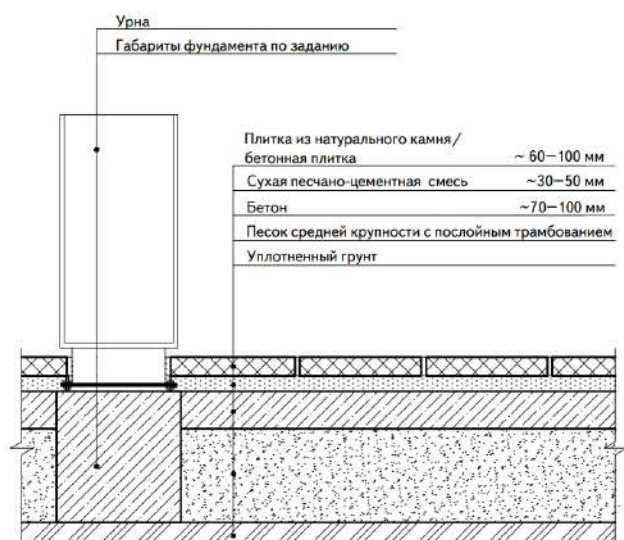
Илл. 5.2.1. ПРИНЦИПИАЛЬНАЯ СХЕМА МОНТАЖА УРНЫ В МОЩЕНИЕ
