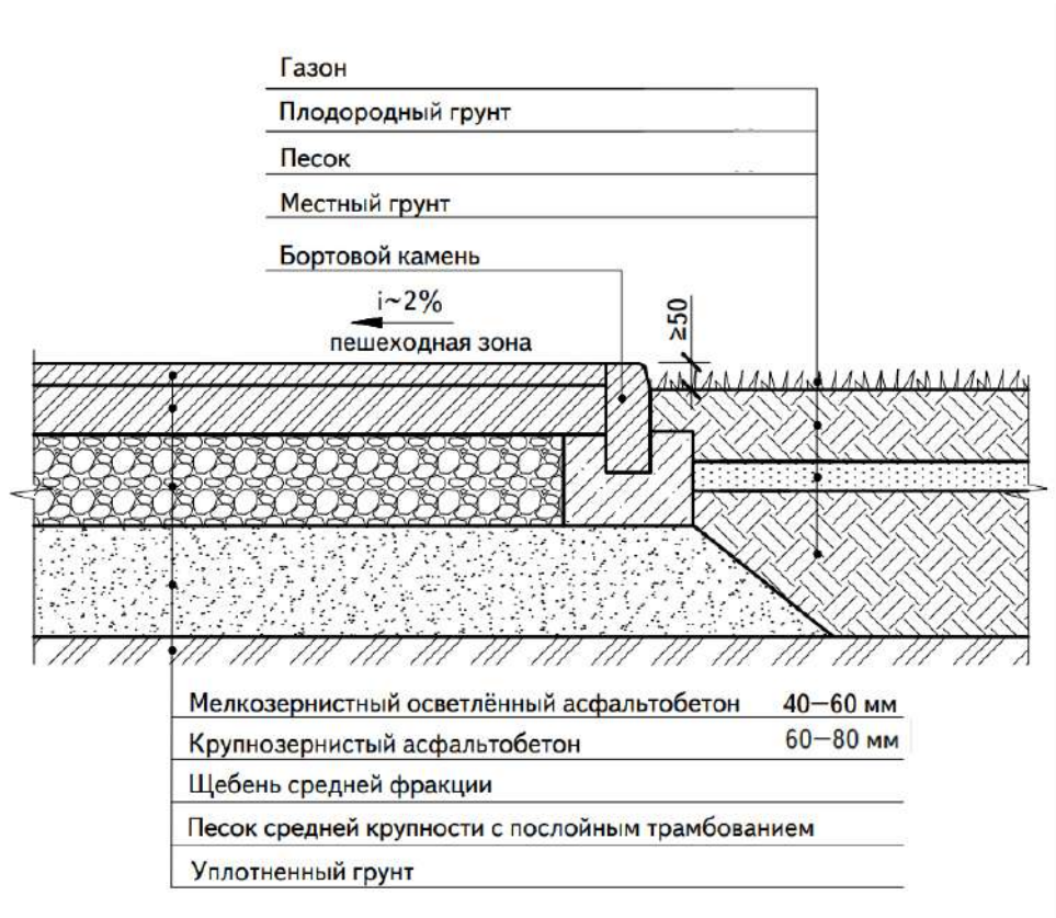
Илл. 1.2.2. Принципиальная схема сопряжения пешеходной зоны из асфальтобетона и газона
