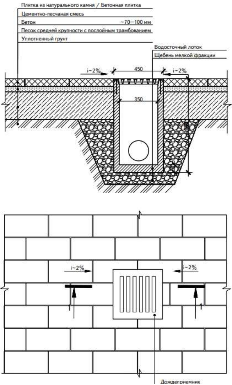
ИЛЛ. 1.2.14. ПРИНЦИПИАЛЬНАЯ СХЕМА УСТРОЙСТВА ДОЖДЕ- ПРИЕМНИКА НА ТРОТУАРЕ
