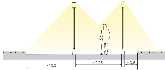
Илл. 4.11. ДВУХРЯДНАЯ ПРЯМОУГОЛЬНАЯ СХЕМА РАСПОЛОЖЕНИЯ ОПОР ОСВЕЩЕНИЯ
