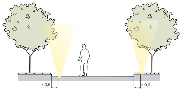
Илл. 3.8. ОСВЕЩЕНИЕ, ВСТРОЕННОЕ В МОЩЕНИЕ
