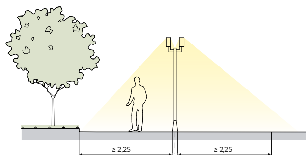
Илл. 4.1.4. ОСЕВАЯ СХЕМА РАСПОЛОЖЕНИЯ ОПОР ОСВЕЩЕНИЯ
