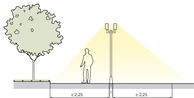
Илл. 6.12. ОСЕВАЯ СХЕМА РАСПОЛОЖЕНИЯ ОПОР ОСВЕЩЕНИЯ
