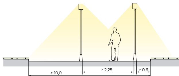
Илл. 4.1.5. ДВУХРЯДНАЯ ПРЯМОУГОЛЬНАЯ СХЕМА РАСПОЛОЖЕНИЯ ОПОР ОСВЕЩЕНИЯ
