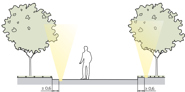
Илл. 5.16. ОСВЕЩЕНИЕ, ВСТРОЕННОЕ В МОЩЕНИЕ
